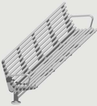
60442 K&K Bank (zeszits) Breedte: 3,15 m Diepte: 0,65 m Totale hoogte: 0,85 m Zithoogte: 0,45 m Van gegritstraald roestvrij staal, met voet voor bevestiging met bodemankers Gewicht: 140 kg
