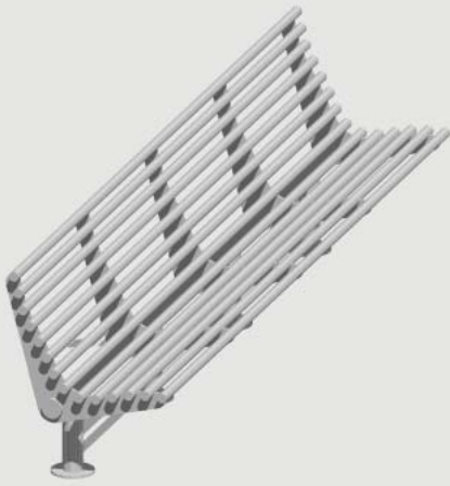
60440 K&K Bank (zeszits) Breedte: 3,00 m Diepte: 0,65 m Totale hoogte: 0,85 m Zithoogte: 0,45 m Van gegritstraald roestvrij staal, met voet voor bevestiging met bodemankers Gewicht: 130 kg
